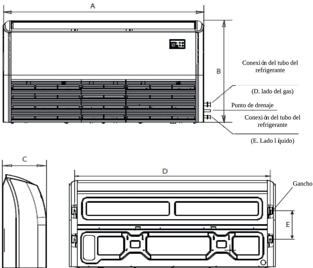
Dimensiones de instalación de las partes interiores
