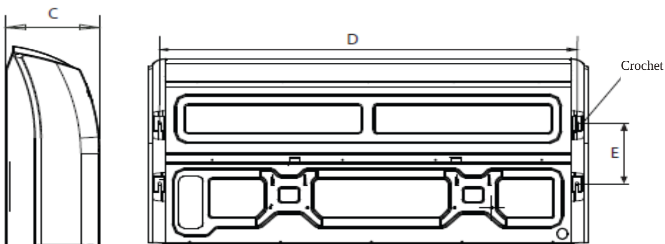
Taille de l'installation des pi èces int érieures
