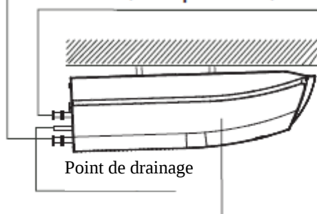
E. Raccordement de la conduite de frigorig  ne (E. C  t   liquide)
