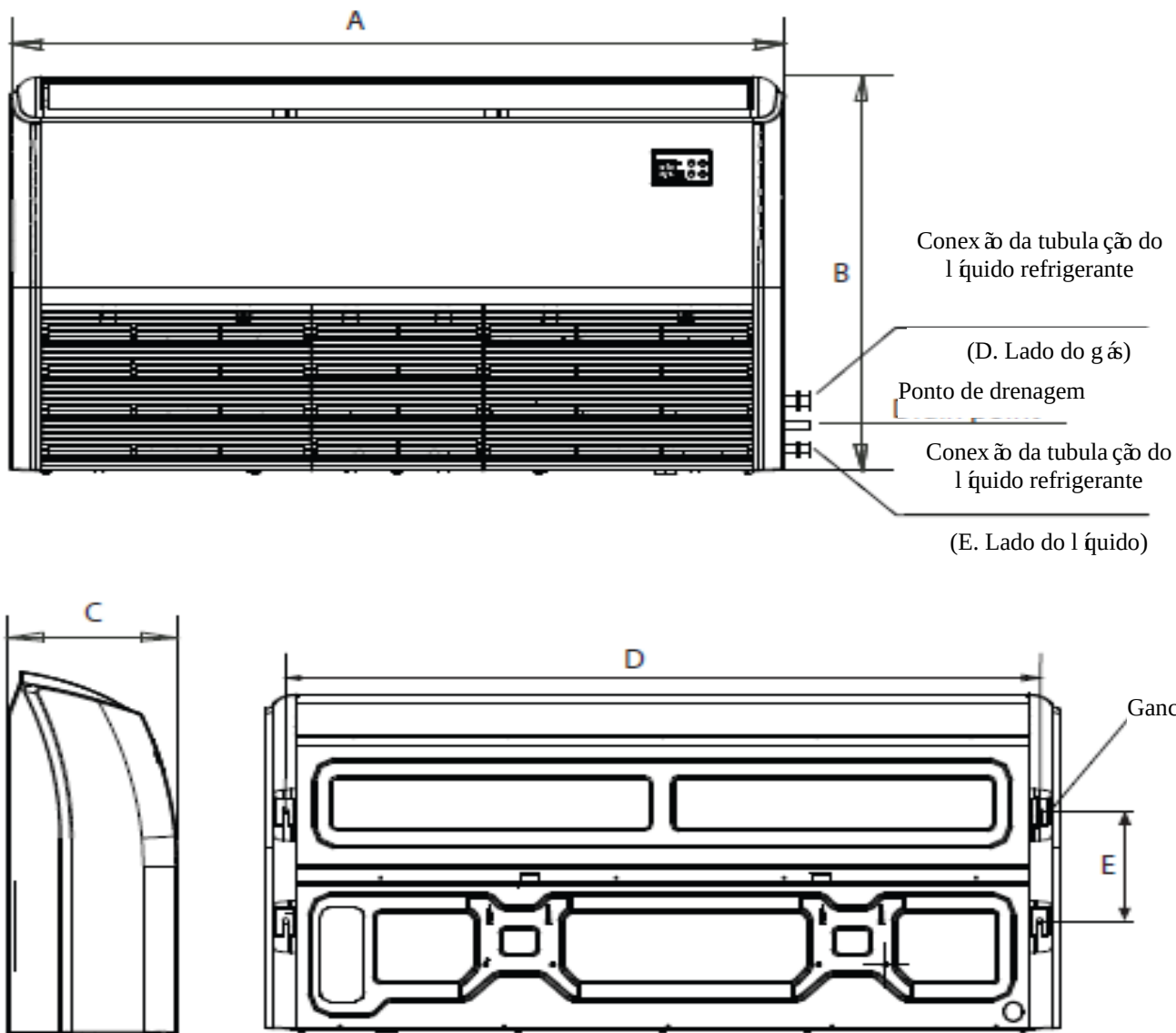
Tamanho de instalação das partes internas
