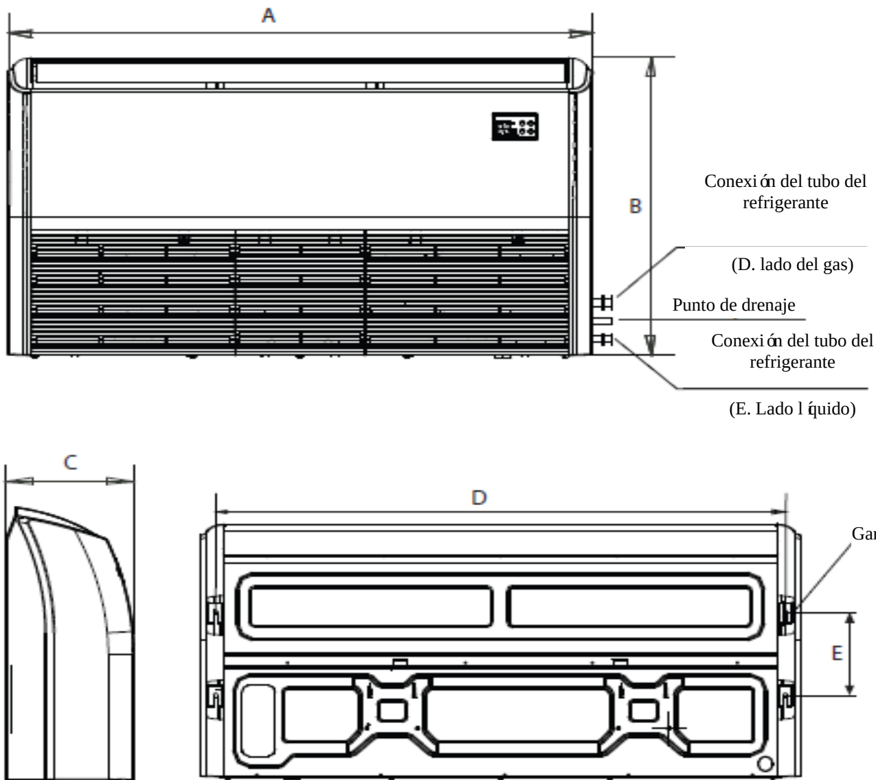
Dimensiones de instalación de las partes interiores
