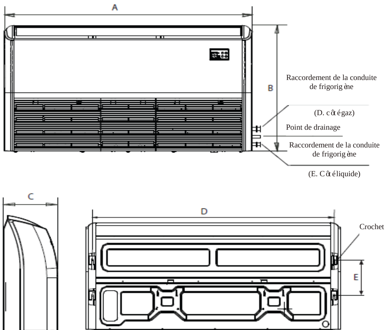
Taille de l'installation des pi èces int érieures
