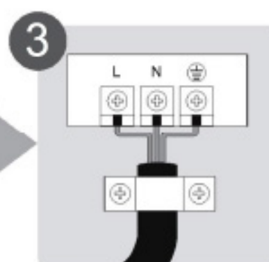
3 Collegare i cavi (Pagina 18)
