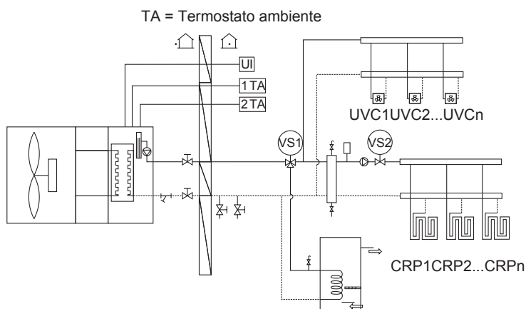
Schema dell'impianto 4
