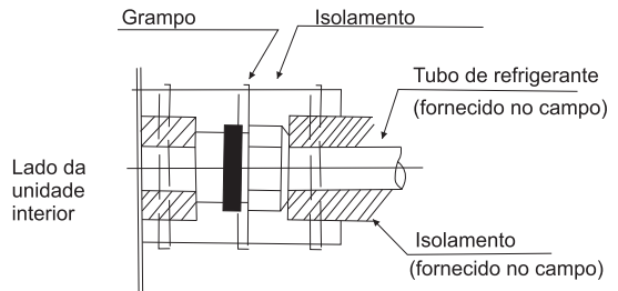
Fig. 4.3 Procedimento de isolamento da tubagem
