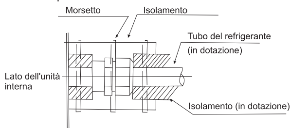
Fig 4.4 Procedura di isolamento dei tubi
