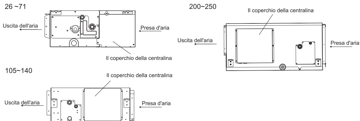
Fig.6.1 Rimuovere le viti sulla centralina.
