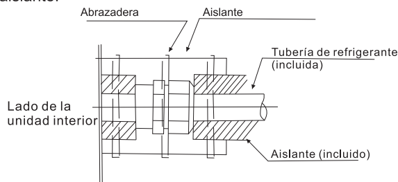
Fig. 4.3 Procedimiento de aislamiento de tuberías
