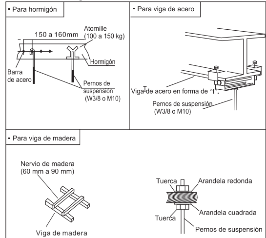
Fig. 3.2.1 Fijar los pernos de suspensión
