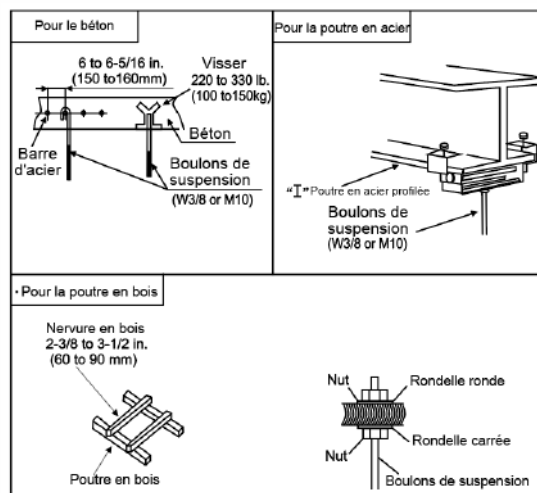
Fig. 3.2.1 Fixation des boulons de suspension
