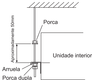
Fig. 3.5 Parafusos e porcas de suspensão
