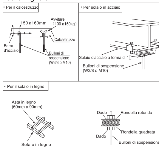
Fig. 3.5 Fissaggio dei bulloni di sospensione 3.2.2 La posizione dei bulloni di sospensione e le tubature
