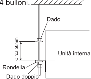
Fig. 3.5 Bulloni e dadi di sospensione
