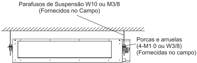
Fig. 3.4 Instalação da unidade interior
