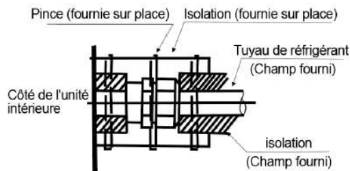
Fig. 4.3 Procédure d'isolation des canalisations
